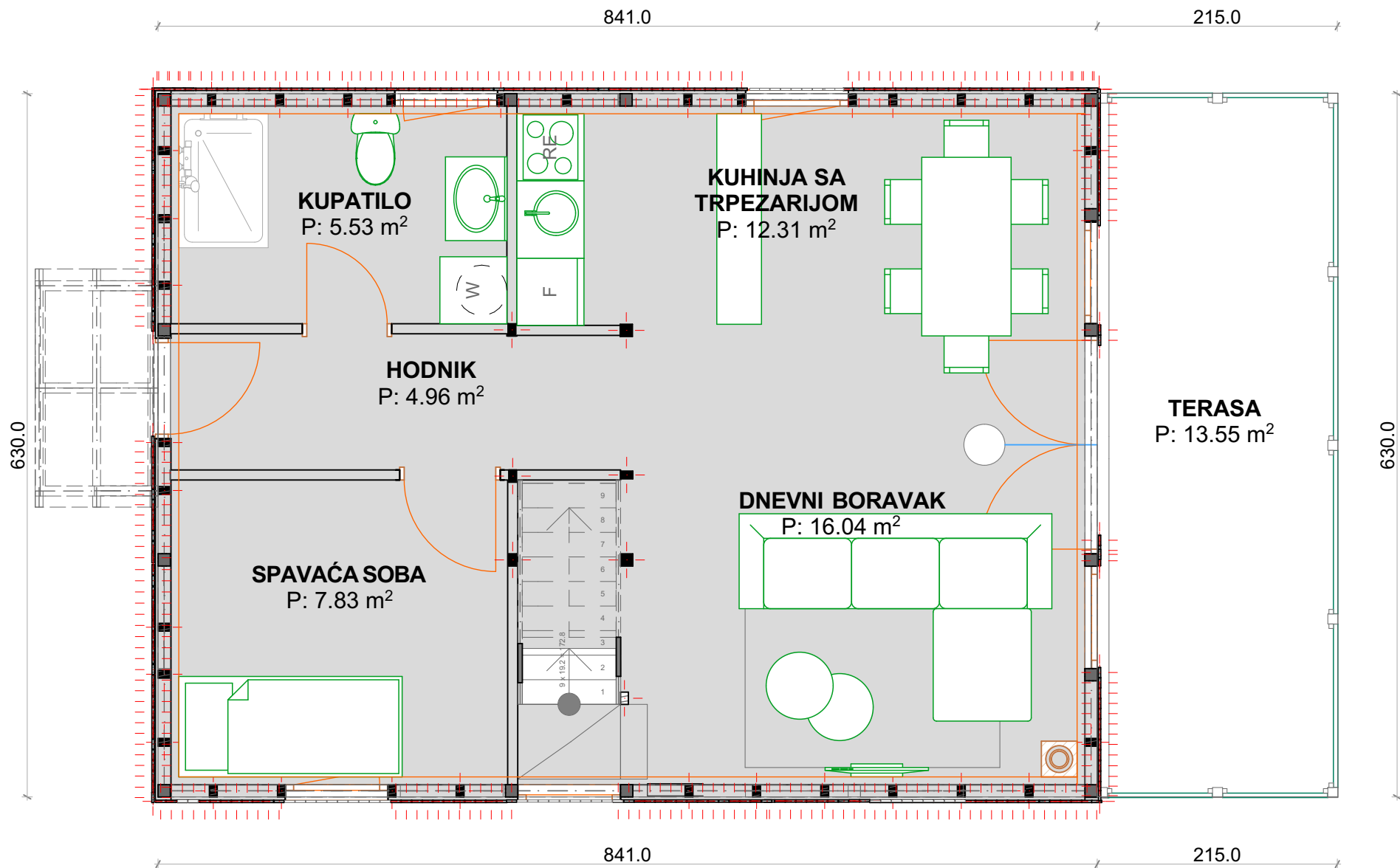
OSNOVA PRIZEMLJA R-1:50
