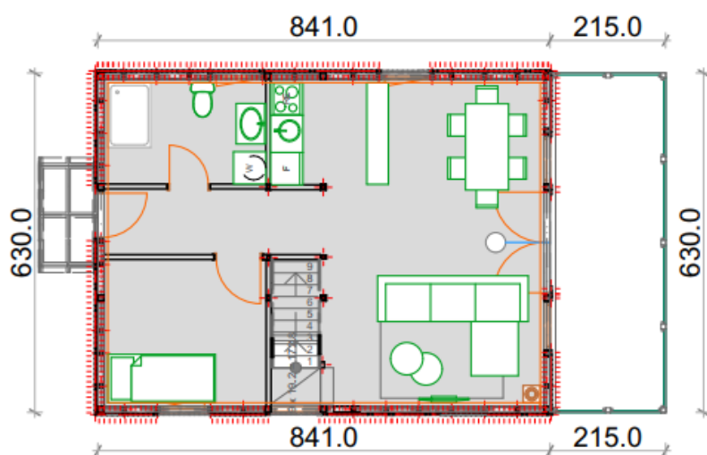
PRIZEMLJE
