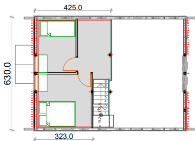
GALERIJA
